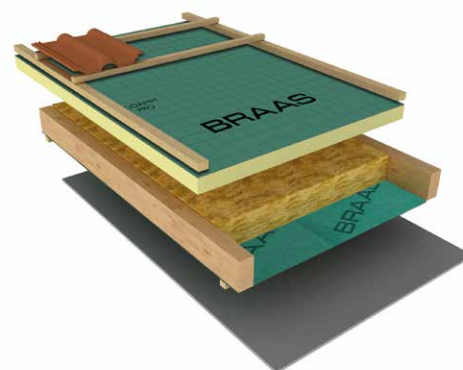
Innenbekleideter Dachstuhl mit DivoDämm Pro über Mineralwolle und DivoDämm Membran 100 2S unter Sparren.
