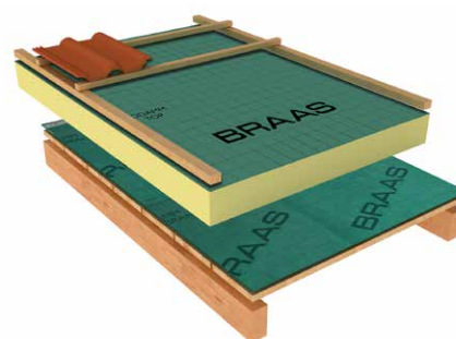
Sichtbarer Dachstuhl mit DivoDämm Top und Dampfsperre DivoDämm Membran 100 2S auf Schalung.
